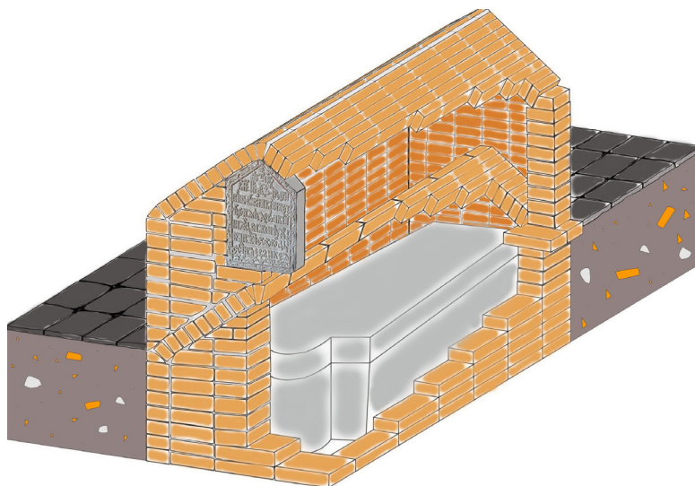
Рис. 15. Кирпичный свод с саркофагом князя Д.М. Пожарского и опирающаяся на него надгробница. Аксонометрическая реконструкция О.А. Тиховой по материалам раскопок 2008 г.
