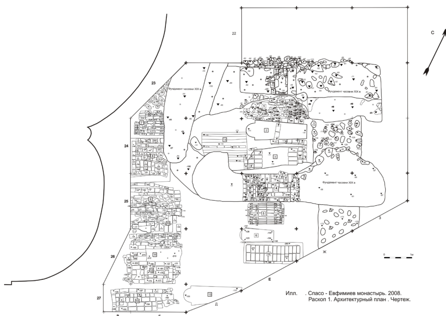
Рис. 11. Уровень склепов и саркофагов в погребальной палатке князей Пожарских и Хованских в Суздальском Спасо-Евфимиевском монастыре. Чертеж О.А. Тиховой.
