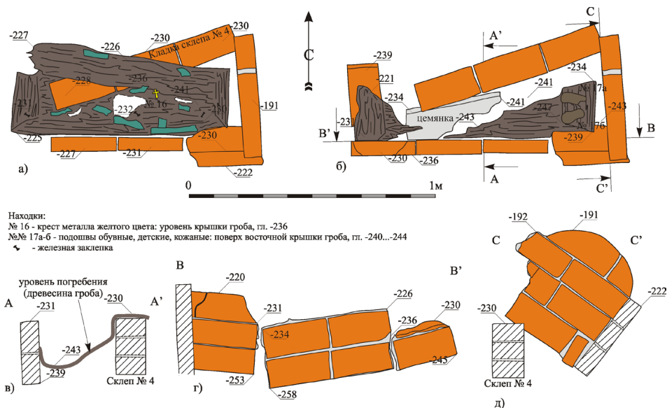
Рис. 12. Два склепа рубежа XVIII–XIX вв. Данилов монастырь, раскопки 2006 г. Обмер и чертеж: С.Г. Шуляев.
