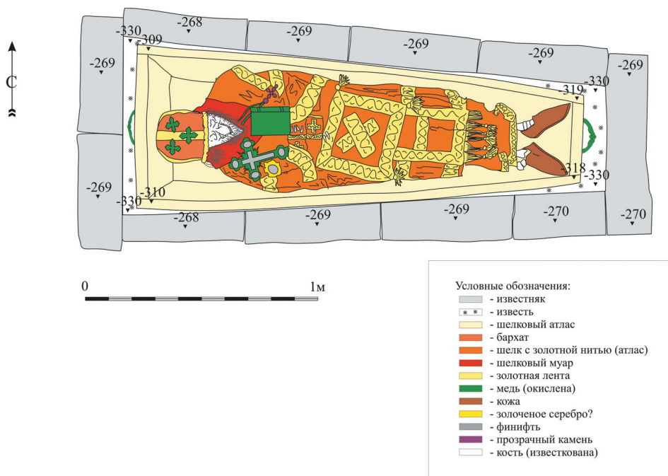
Рис. 13. Погребение архиепископа Никифора (Феотоки), 1800 г. Данилов монастырь, раскопки 2006 г. Обмер и чертеж: С.Г. Шуляев.
