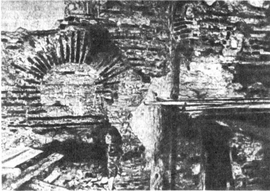
Работы по изучению кладок Полоцкой Софии XI в. (По Н. Кайгородову)
